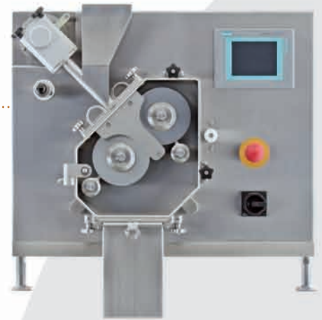
KOMPAKTIERBETRIEB DURCHSATZ BIS ZU 20 kg/h
